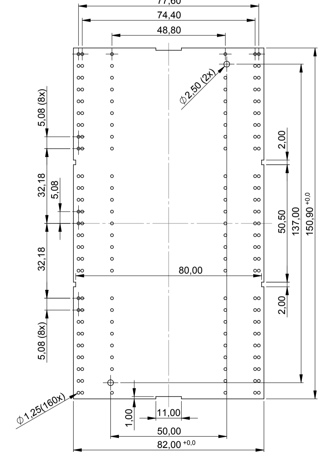
Leiterplatte für das Unterteil Raster 5.08 PCB for base block 5.08
