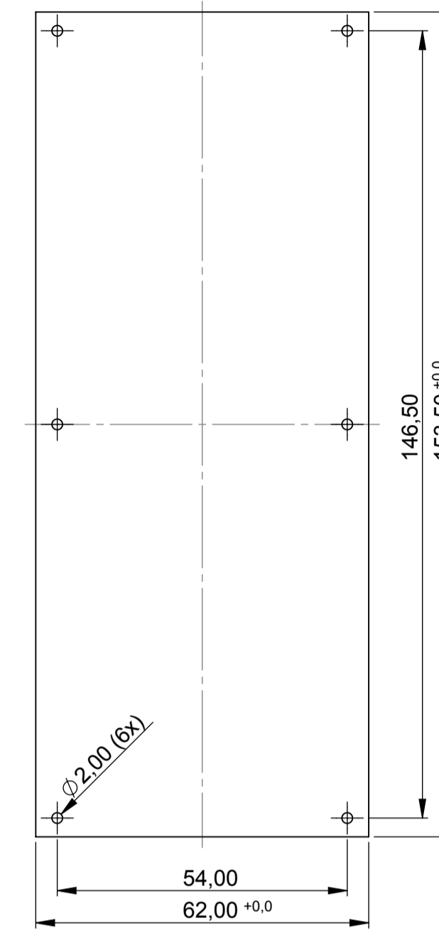
Platine Oberteil PCB top
