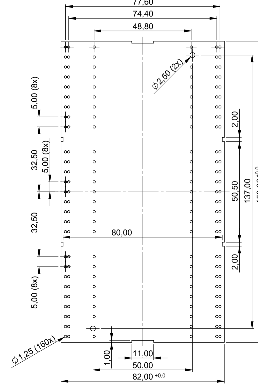
Leiterplatte für das Unterteil Raster 5.0 PCB for base block 5.0
