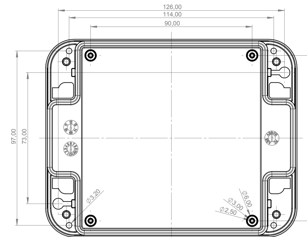
Oberenteil Innenansicht Top part inside view
